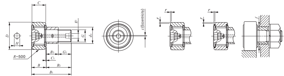
CFE ... VBR Außendurchmesser des Exzenterings d_e 16-41mm
