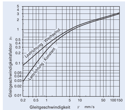
Abb. 3 Gleitgeschwindigkeitsfaktor
