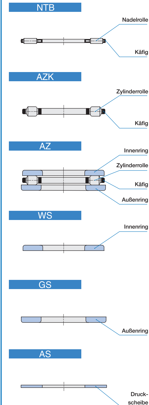
Aufbau von Axiallagern
