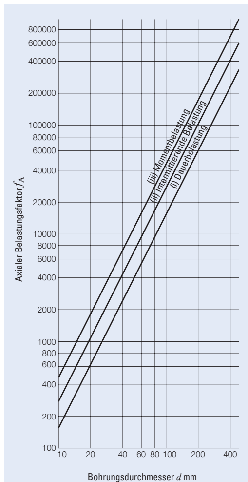
Abb. 1 Axialer Belastungsfaktor
