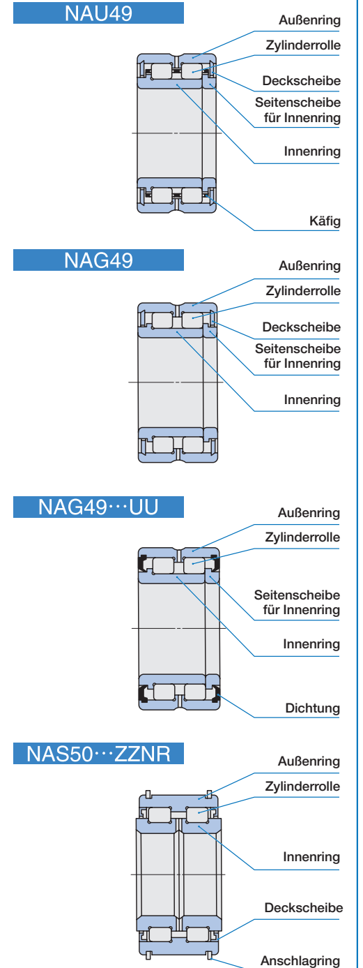
Aufbau von Zylinderrollenlagern
