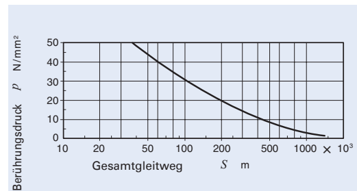
Abb. 6 Berührungsdruck und gesamter Gleitweg für wartungsfreie PILLOBALL-Gelenkköpfe
