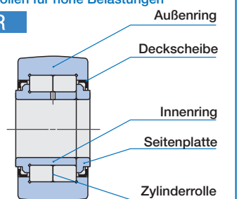
Aufbau von Stützrollen für hohe Belastungen
