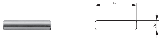
Rollendurchmesser 1 – 6mm
