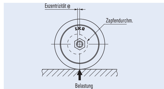
Abb. 3 Referenzposition zur Einstellung von Kurvenrollen mit festem Exzenterspindel und Kurvenrollen mit Exzenterring
