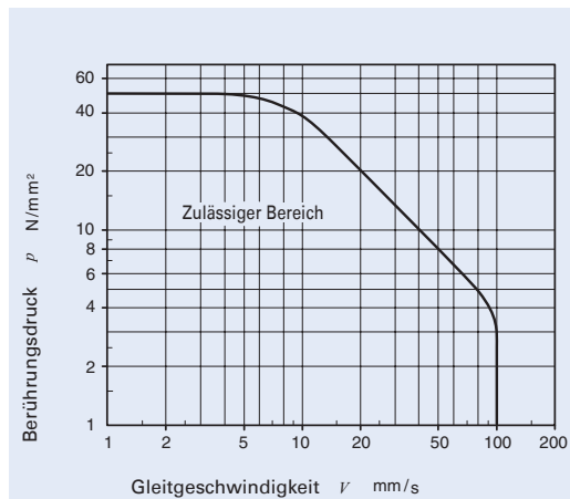
Abb. 2 pV Diagramm für wartungsfreie PILLOBALLs
