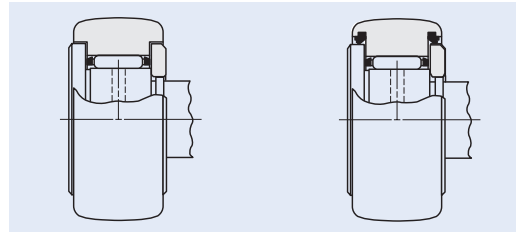
«Mit Deckscheibe»
