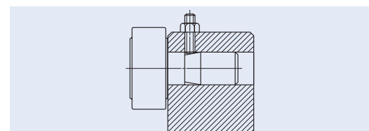
Abb. 6 Montagebeispiel für einfach zu montierende Kurvenrollen
