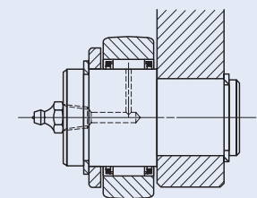
Abb. 3 Beispiel für den Einbau einer Stützrolle ohne Innenring
