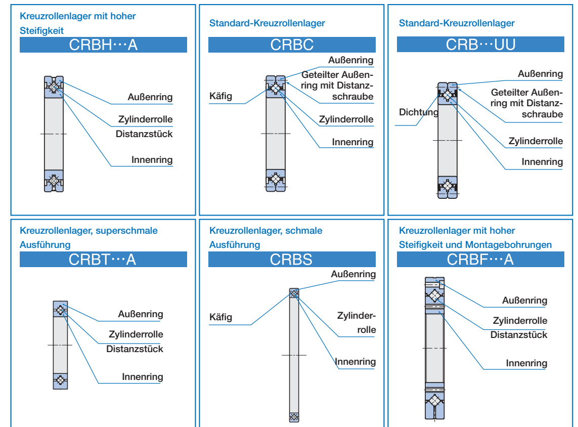
Aufbau von Kreuzrollenlager
