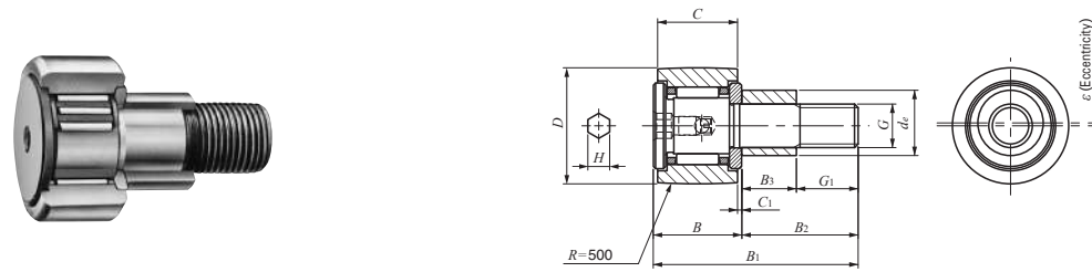
CFE...BR Außendurchmesser des Exzenterrings d_e 9-13mm
