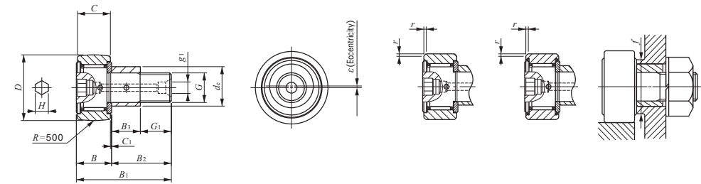
CFE...BR Außendurchmesser des Exzenterrings d_e 16-41mm
