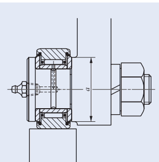
Abb. 1 Kontaktmaß „a“
