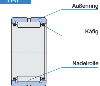
Aufbau der Nadellager ohne/mit Innenring, abgedichtet
