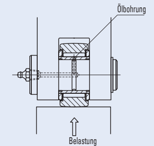
Abb. 2 Lage der Ölbohrung und Belastungsrichtung
