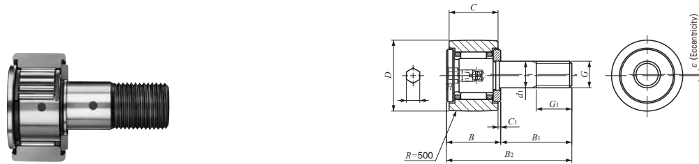
CFES...BR Zapfendurchm. d_1 6-10mm
