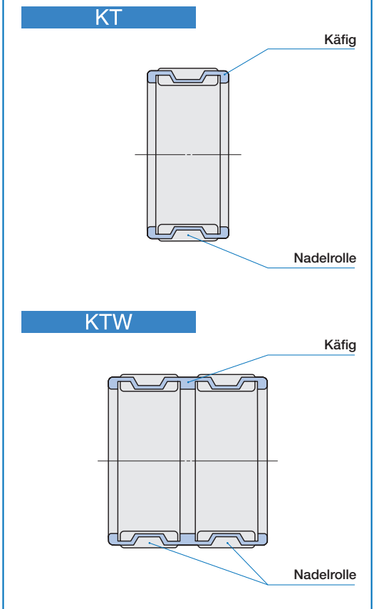
Aufbau von Nadelkränzen für allgemeine Anwendung
