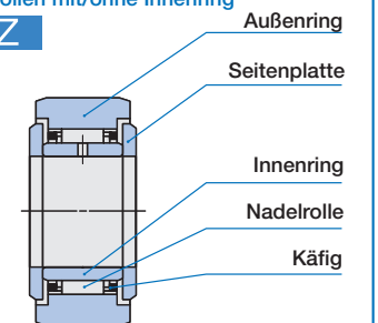
Aufbau von Stützrollen mit/ohne Innenring
