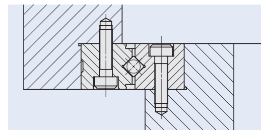
Abb.4 Beispiel für die Montage am Gehäuse des Kreuzrollenlagers mit hoher Steifigkeit und Montagebohrungen
