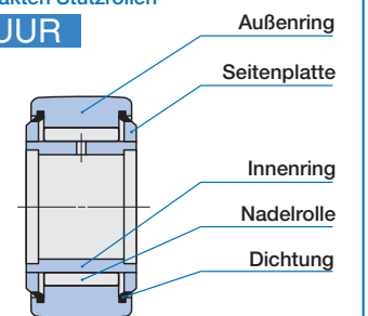
Aufbau von kompakten Stützrollen
