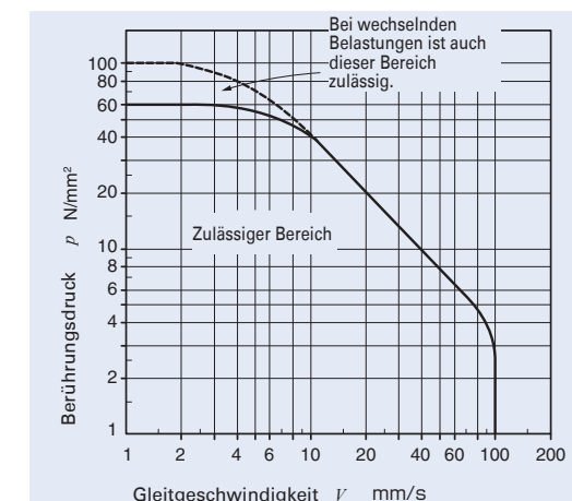
Abb. 1 pV -Diagramm für Stahl/Stahl/Gelenklagern
