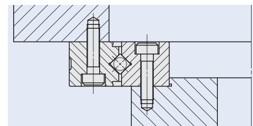
Abb.3 Beispiel für die direkte Montage an der Kontaktfläche des Kreuzrollenlagers mit hoher Steifigkeit und Montagebohrungen
