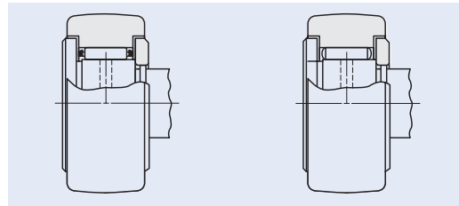
«Mit Käfig»
