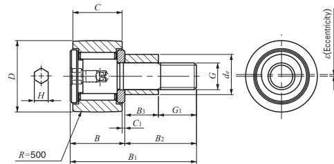
CFE ... VBR Außendurchmesser des Exzenterings d_e 9-13mm
