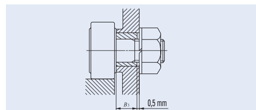
Abb. 5 Länge der Montagebohrung bei Kurvenrollen mit Exzenterring
