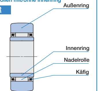
Aufbau von Stützrollen mit/ohne Innenring
