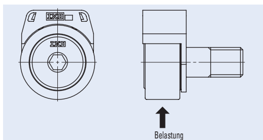
Abb. 8 Lastrichtung der Kurvenrolle
