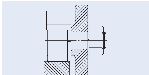
Abb. 7 Montage der C-Lube-Einheit
