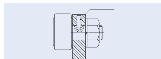
Abb. 4 Beispiel für den Einbau einer Kurvenrolle mit festem Exzenterspindel
