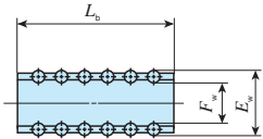
Ball cage
