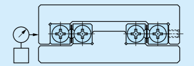
Abb. 31 Beispiel zum Einstellen der Vorspannung
