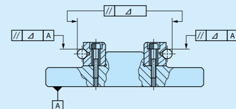
Abb. 28 Genauigkeit der Führungsmontage
