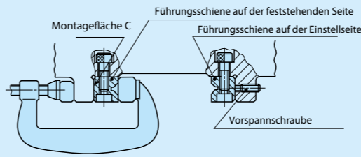
Abb. 29 Führungsmontage auf der Tischseite
