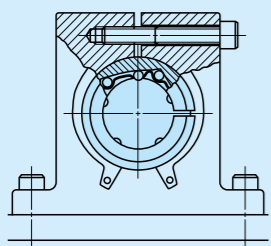
Abb. 2 Beispiel für Spieleinstellung
