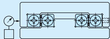
Abb. 24 Beispiel zum Einstellen der Vorspannung
