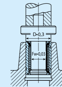
Abb. 5 Presspassung der Buchse
