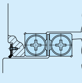
Abb. 8 Beispiel für Abstreifer
