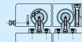
Abb. 6 Montagebeispiel
