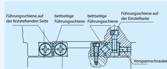
Abb. 26 Montagebeispiel für eine Standardausführung der CRW-Baureihe
